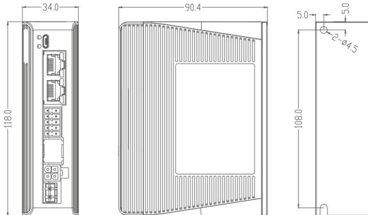
图 2-2 DM3C-522/556/870 安装尺寸图(单位：mm)
