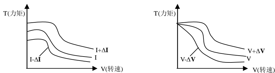
图 6 矩频特性图
