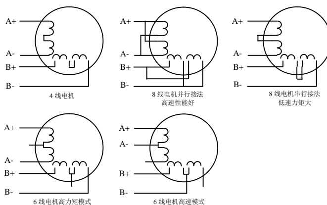
图 7 电机接线图
