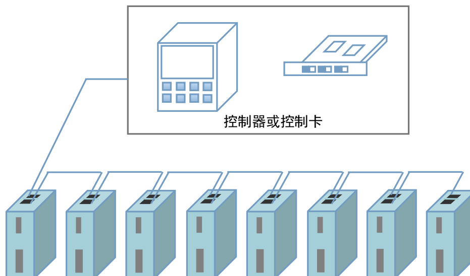
图 7 DM556-CAN 接线示意图（最后一个驱动器 SW8 设置为 on）
