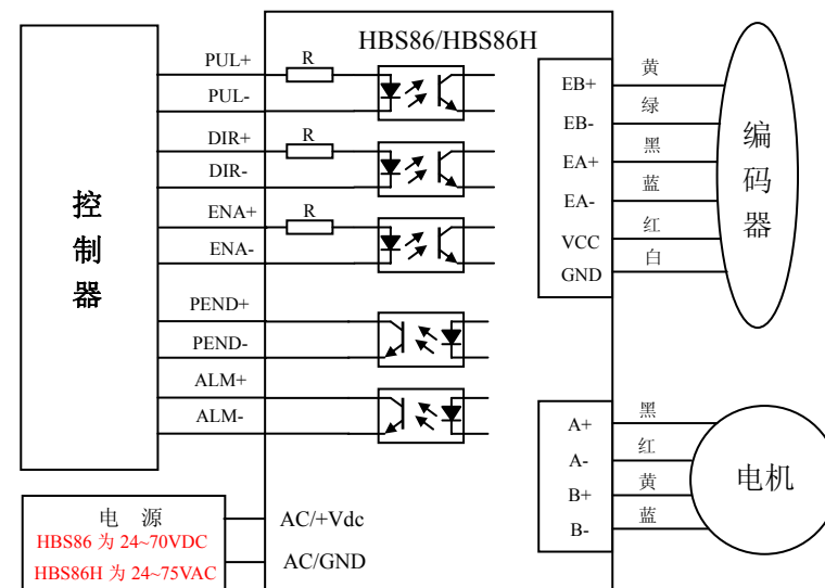
图 7 典型接线图
