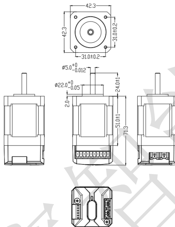
图 2-1 IDM42-RS06 智能一体式步进电机的机械尺寸
