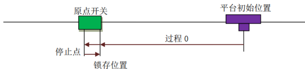
图 4.7 点锁存回零方式示意图
