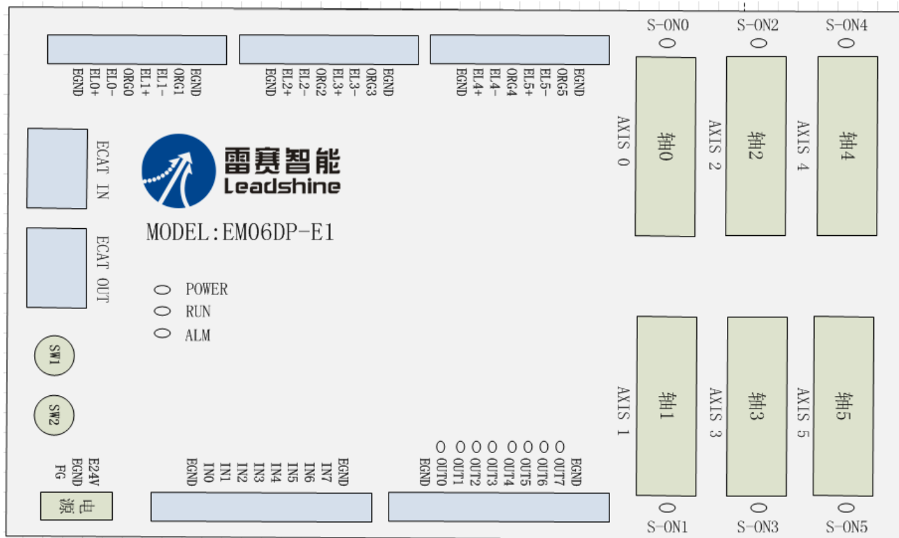
图 2.2 EM06DP-E1 定位模块接口示意图
