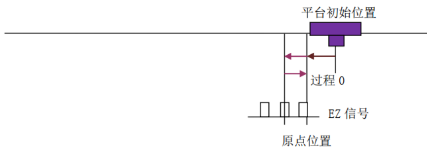
图 4.9 单独记一个 EZ 锁存回零方式示意图
