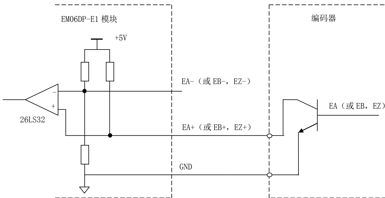
图 2.11 编码器单端接线方式图
