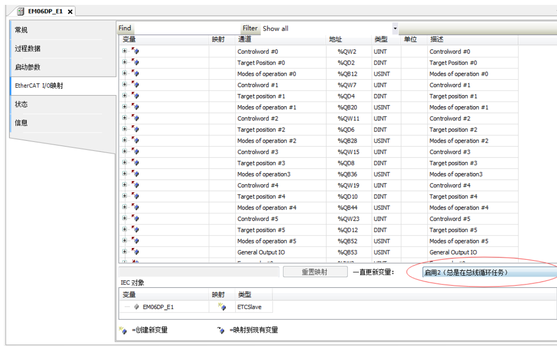
图 6.16 从站 I/O 映射配置界面
