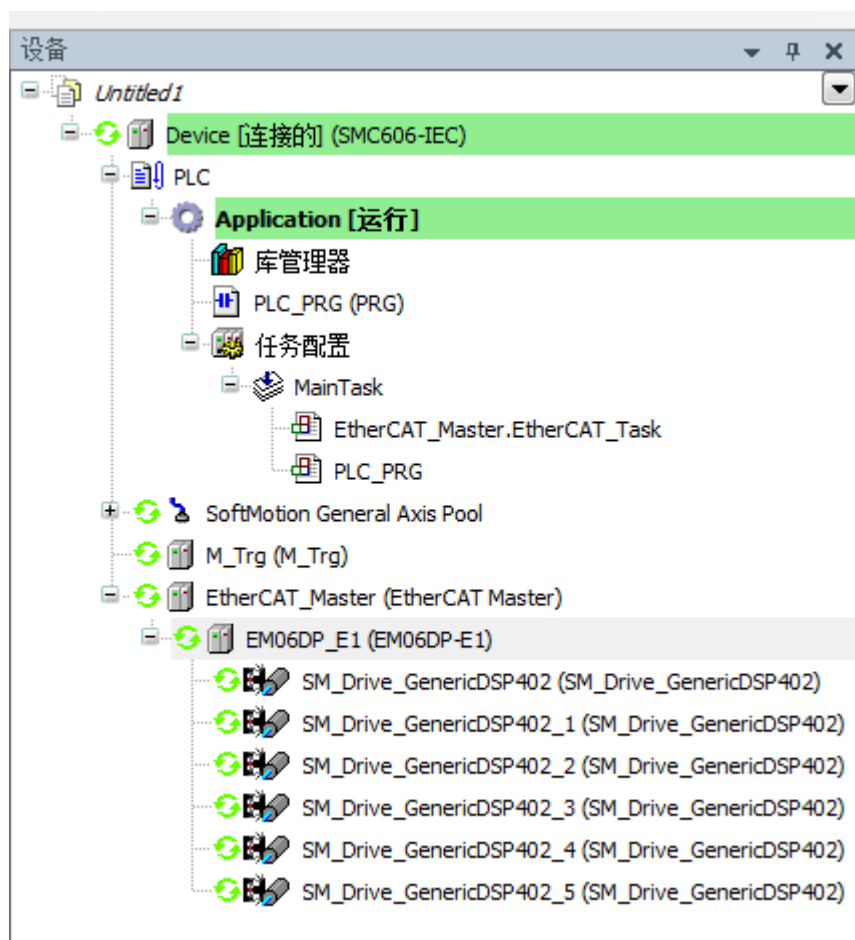
图 6.14 添加从站完成
