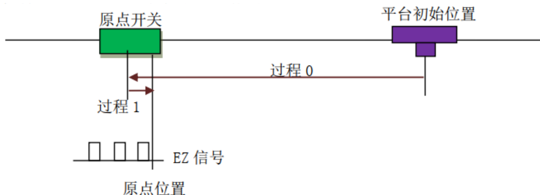
图 4.6 一次回零再反找 EZ 信号回零方式示意图
