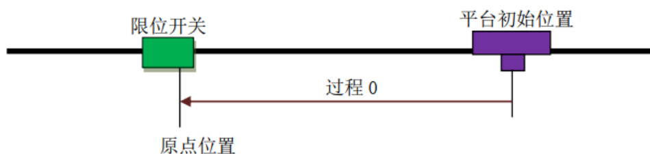
图 4.11 一次限位回零方式示意图
