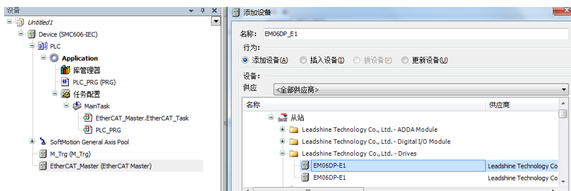
图 6.10 添加 EM06DP-E1 模块
