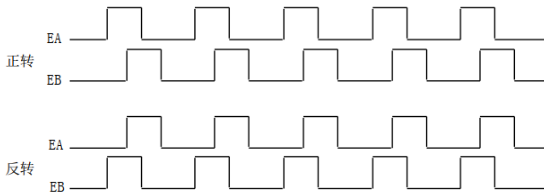
图 4.7 A/B 相正交信号
