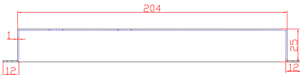
图 1.2 正视图
