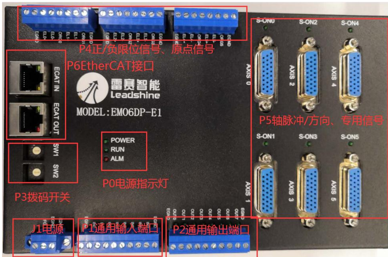
图 2.2 EM06DP-E1 定位模块接口分布图
