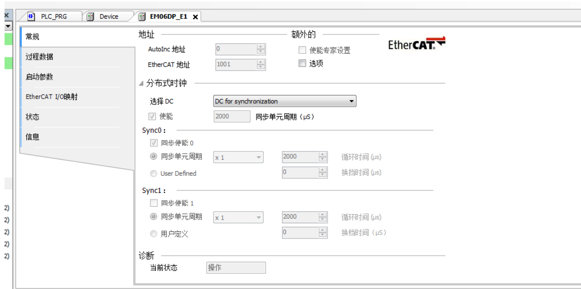
图 6.15 EM06DP-E1 参数配置界面
