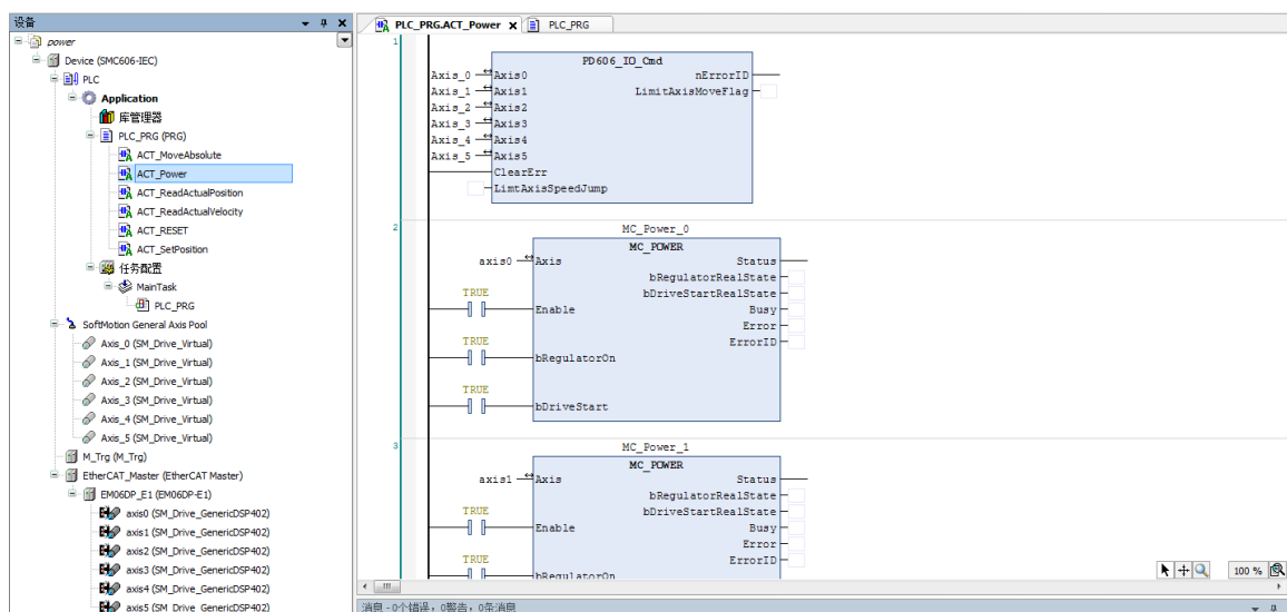
图 6.20 上电模块
