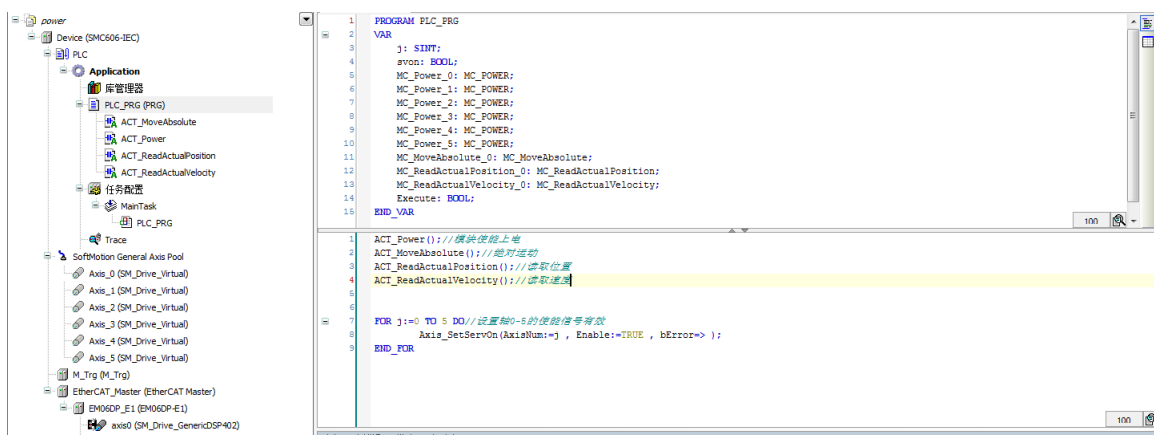
图 6.24 主程序逻辑
