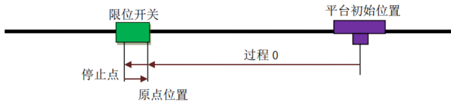
图 4.12 一次限位回零加回找回零方式示意图
