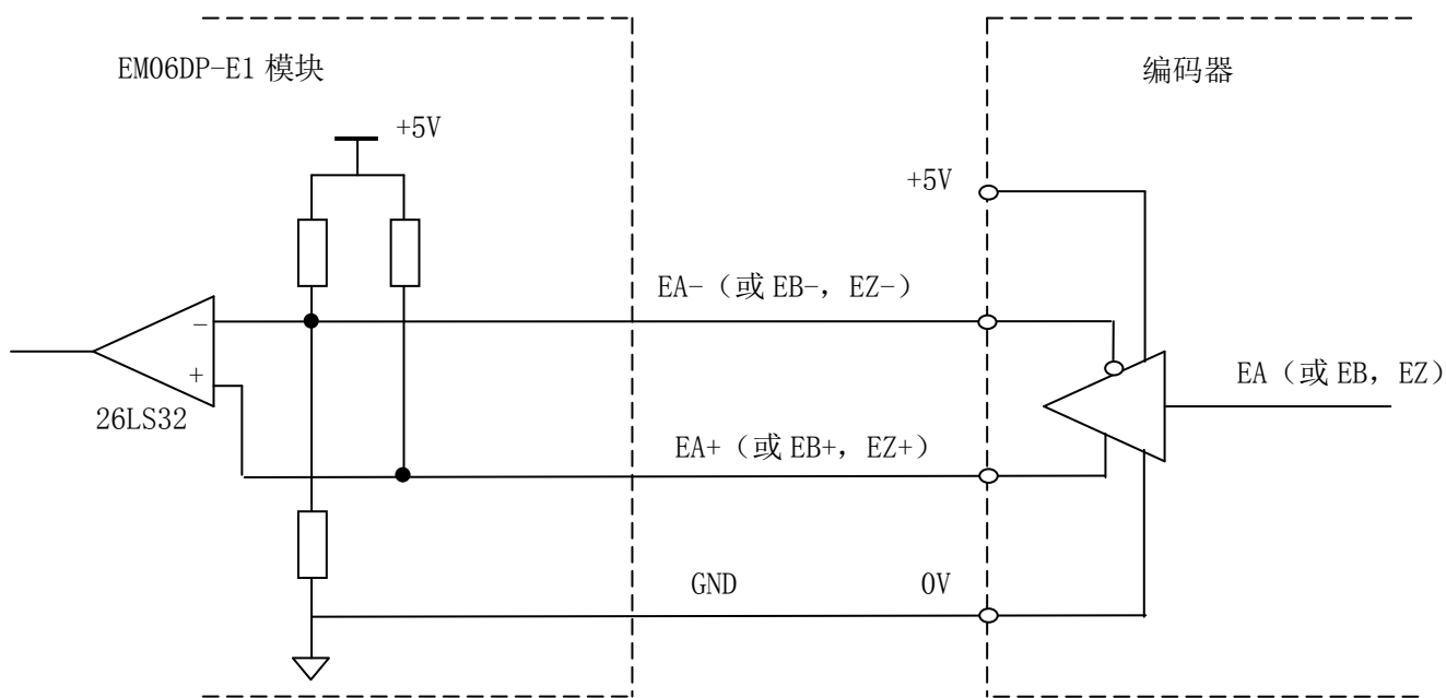
图 2.10 编码器差分接线方式图
