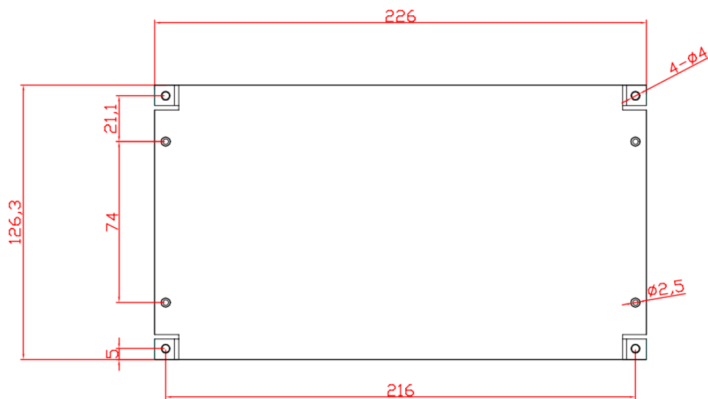
图 1.1 俯视图
