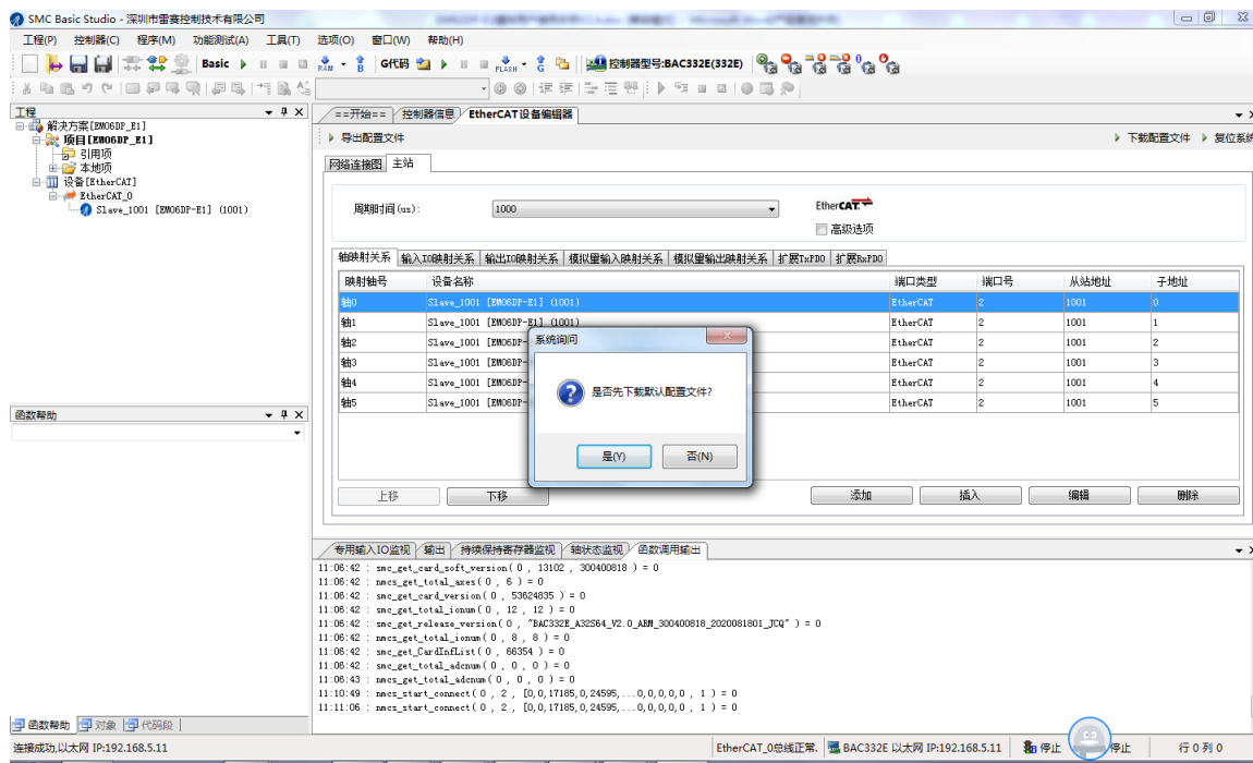
图6.34 自动扫描设备
