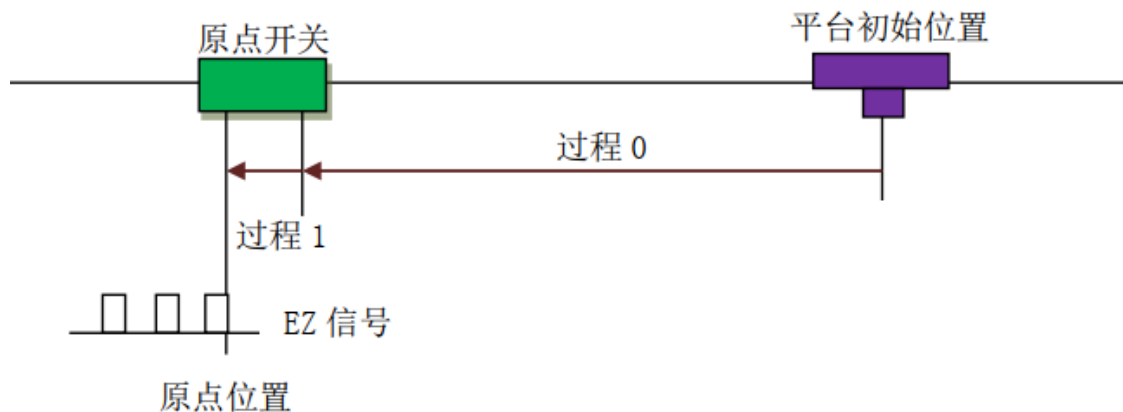
图 4.8 原点锁存加同向 EZ 锁存回零方式示意图
