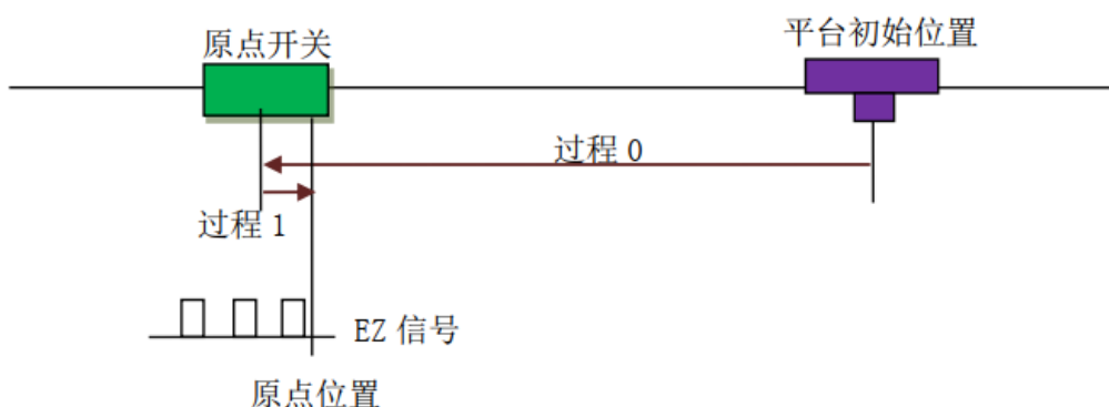
图 4.10 原点锁存加反向 EZ 锁存回零方式示意图
