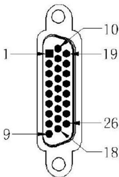
图 5-2 DB26 端子示意图
