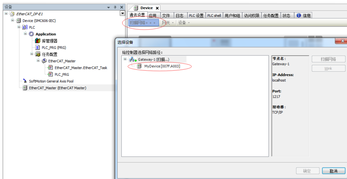
图 6.11 扫描网络
