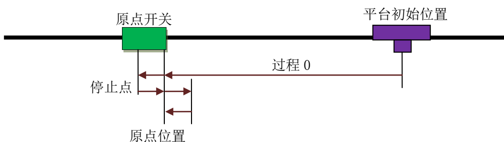
图 4.3 二次回零方式示意图
