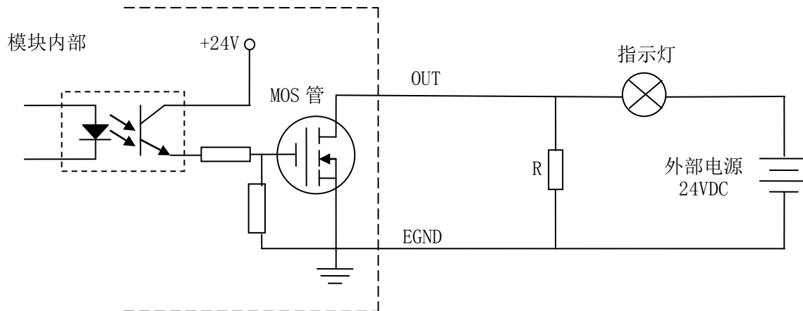
图 2.3.3 通用输出接线图
