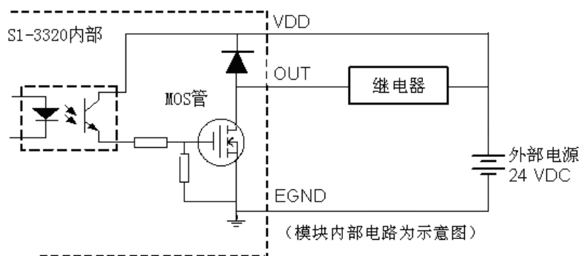
图 2.7 接小型继电器的原理图
