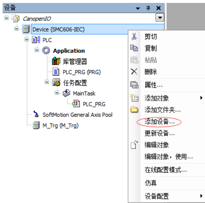
图 4.1 添加设备
