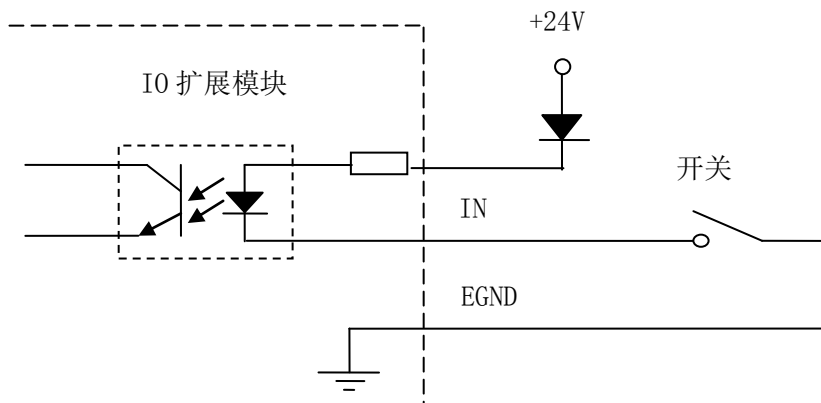
图 2.4 输入接口接线图
