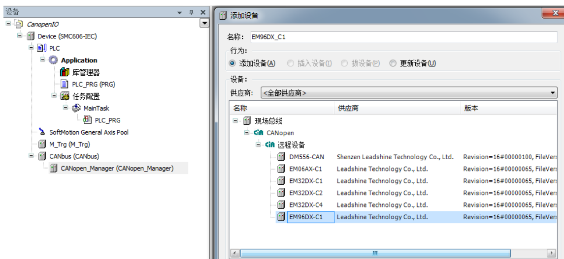
图 5.7 添加 EM96DX-C1 模块
