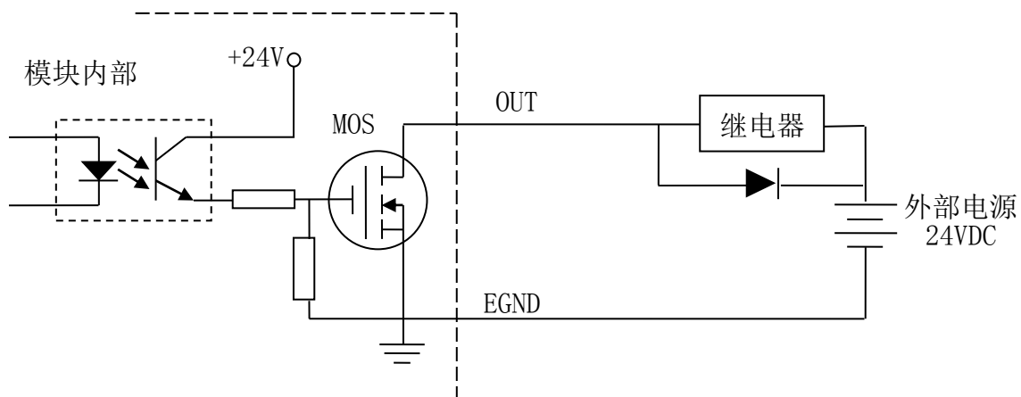
图 2.11 通用输出接线图
