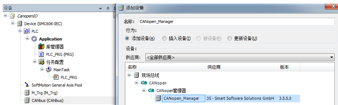
图 5.4 添加 CANopen 设备
