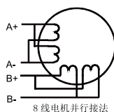
8线电机并行接法 高速性能好
