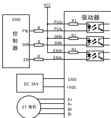
共阳极接法
