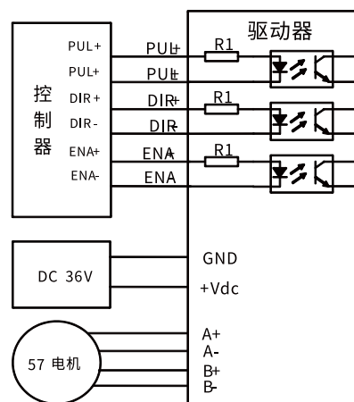
差分接法
