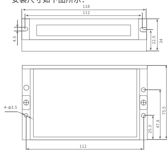
DM556(V3.0)/DM870(V3.0)/3DM580S安装尺寸图（单位：mm）
