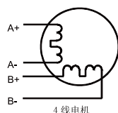
4线电机
