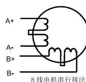
8线电机串行接法 低速力矩大
