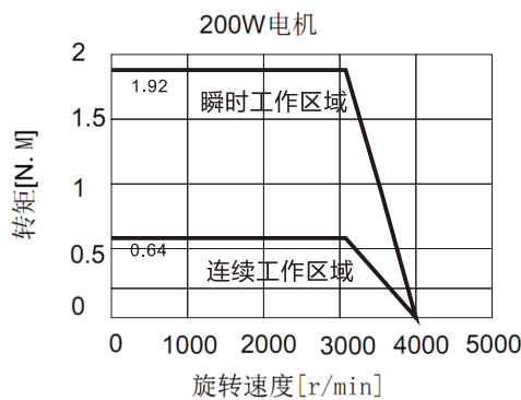
③ 200W电机力矩曲线
