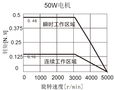
③ 50W电机力矩曲线
