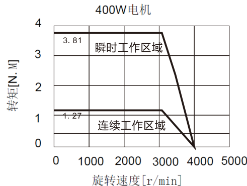
④ 400W电机力矩曲线
