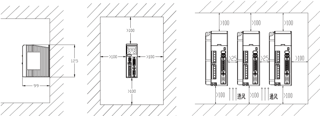
单台驱动器安装间隔
