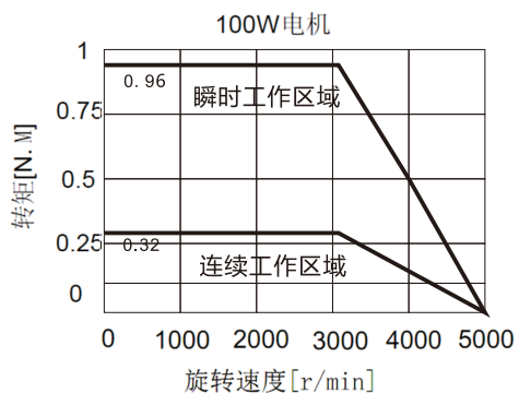
④ 100W电机力矩曲线
