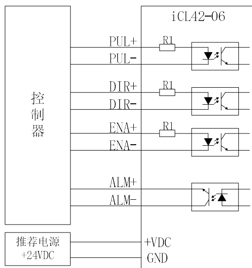
图 4 典型接线图
