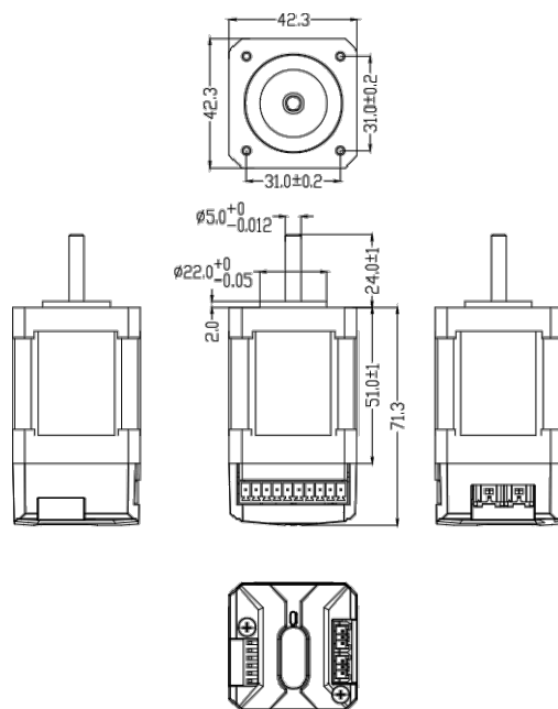
图 1 iCL42-06 安装尺寸图
